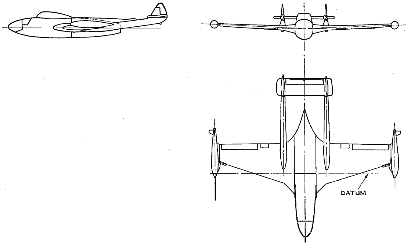
FIG. 1. Sea Venom .
