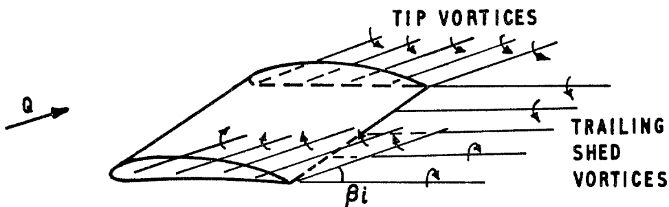
(B) TIP VORTEX METHOD
