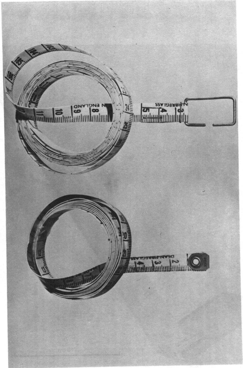
FIG. 14. Glass-cloth tapes.
